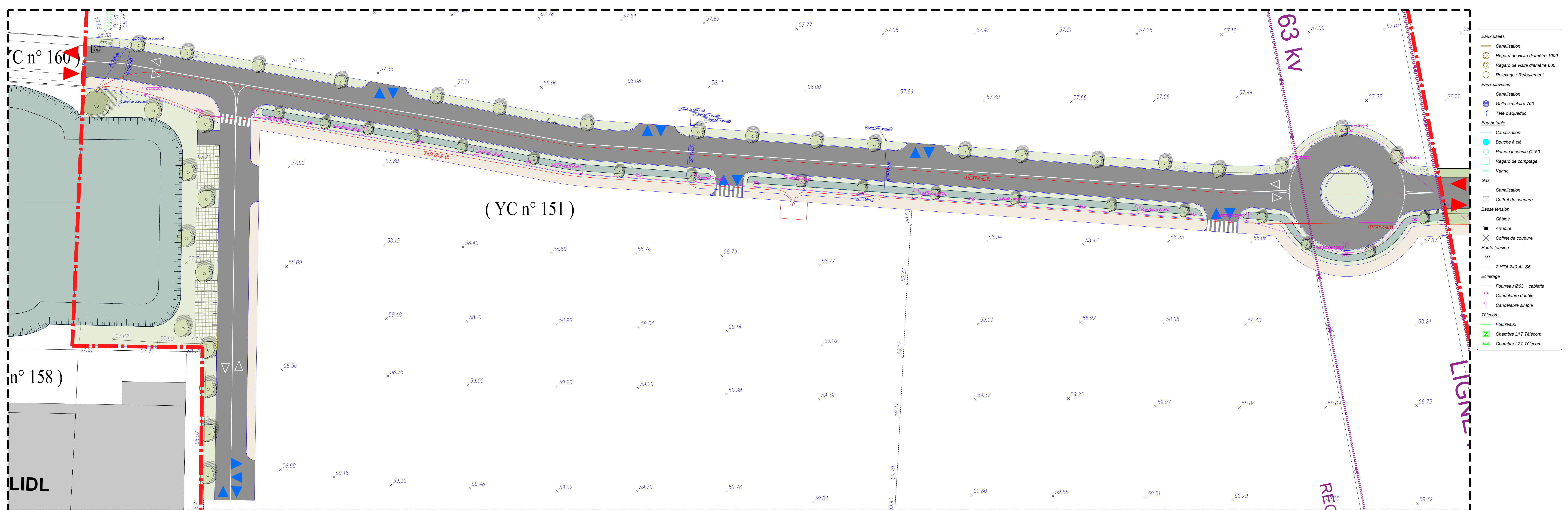
ZOOM VOIRIE COMMUNE Echelle : 1 / 300
